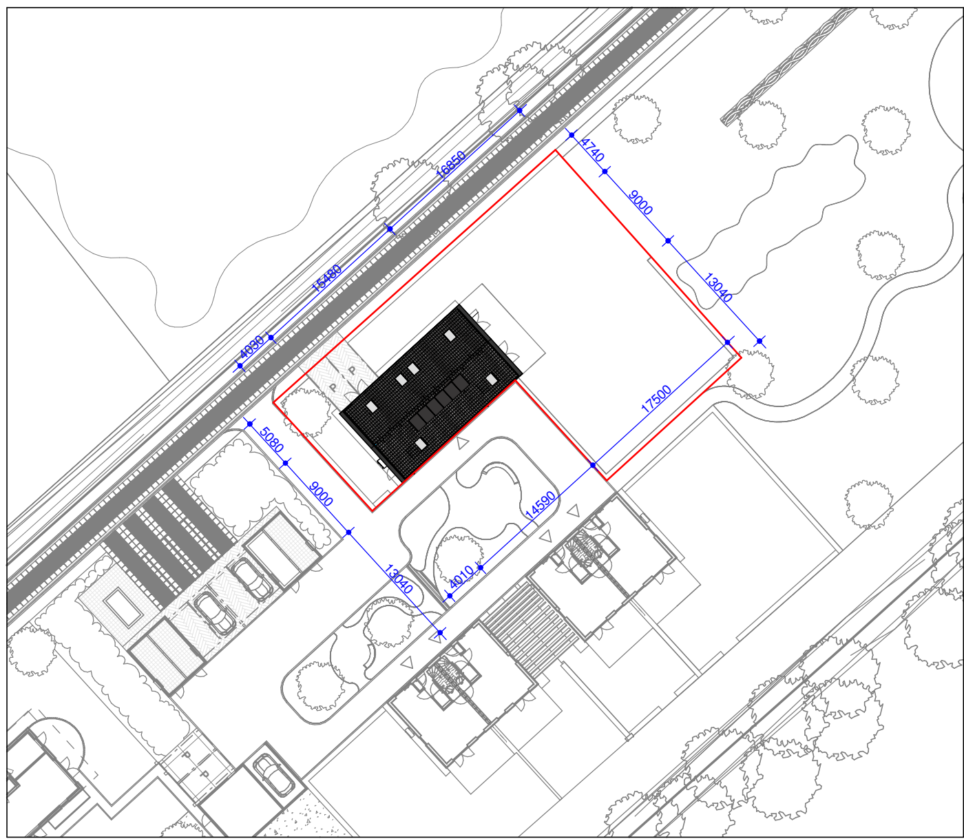
Situatie 1 : 500
