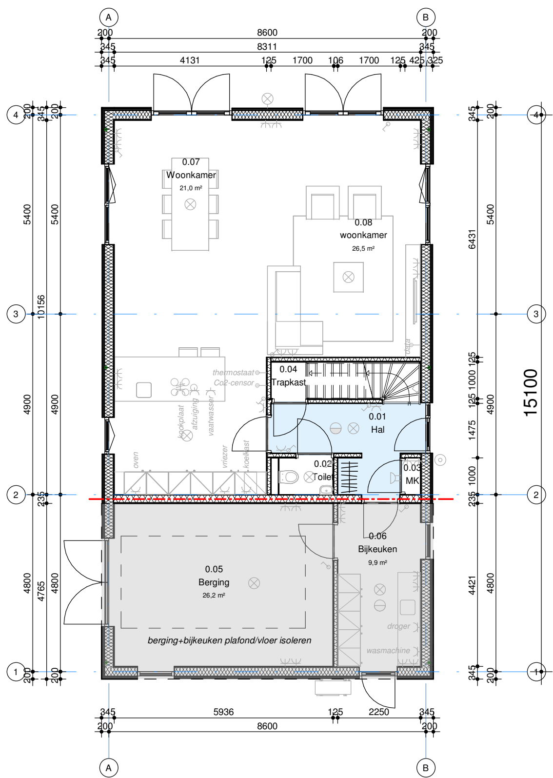
begane grond 1 : 100
