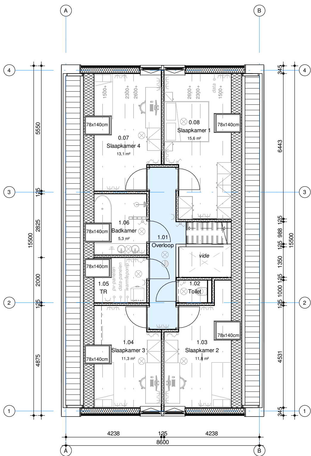
eerste verdieping 1 : 100
