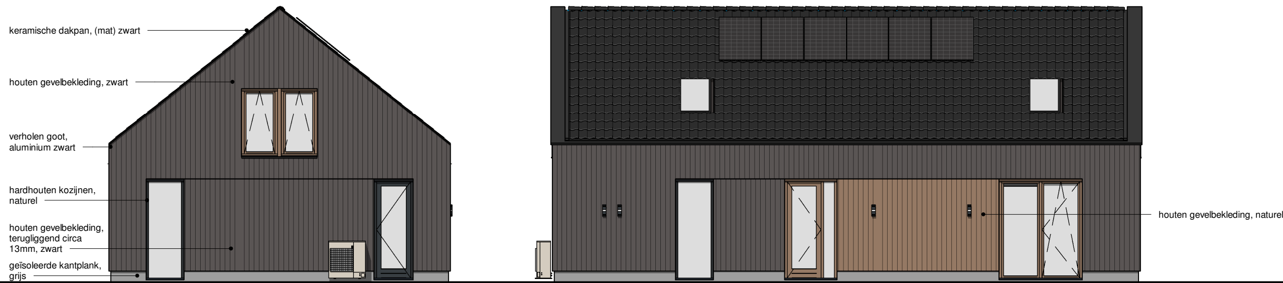
vooraanzicht 1 : 100
