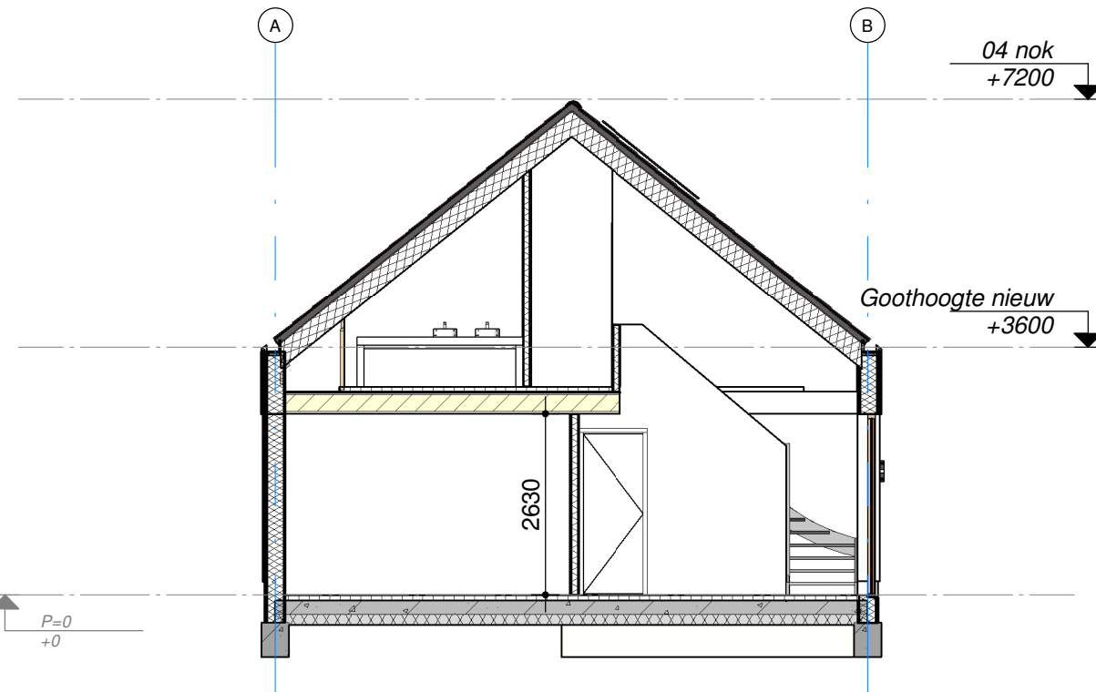
Doorsnede 1 : 100
